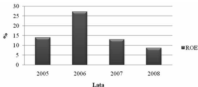
Wykres 2. Rentowność kapitału własnego badanej grupy kapitałowej w latach 2005–2008
