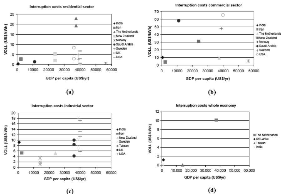
Rys. 1. Porównanie wartości VOLL dla różnych krajów dla sektora gospodarstw domowych (a), usług (b), przemysłu (c) oraz gospodarki jako całości (d). Koszty zostały wyrażone na kWh niedostarczonej energii.
